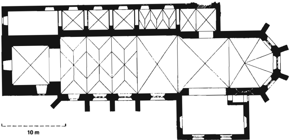
Abb. 2: Grundriß der Herzebrocker Kirche um 1900 (nach Bau- und Kunstdenkmäler von Westfalen: Kreis Wiedenbrück 1901 S. 32).
